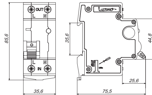
Рис. 3. Размеры УЗДП
